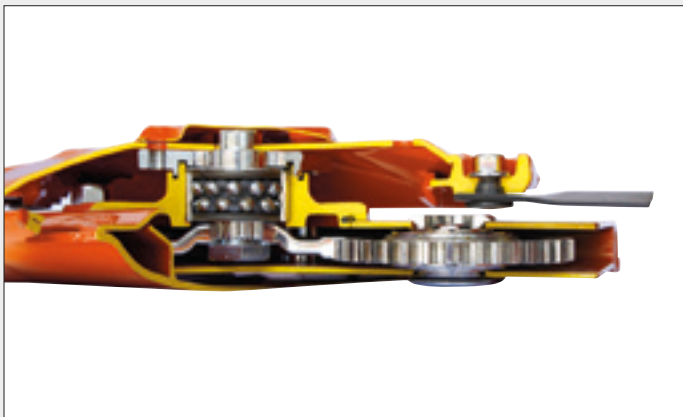
Messerbefestigung durch Bolzen
